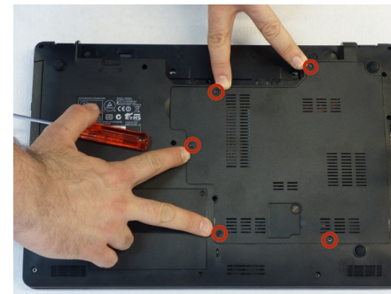
Entfernen Sie 5 Schrauben und Sie haben Zugriff auf die wichtigsten Komponenten des Laptop why! W253EU
